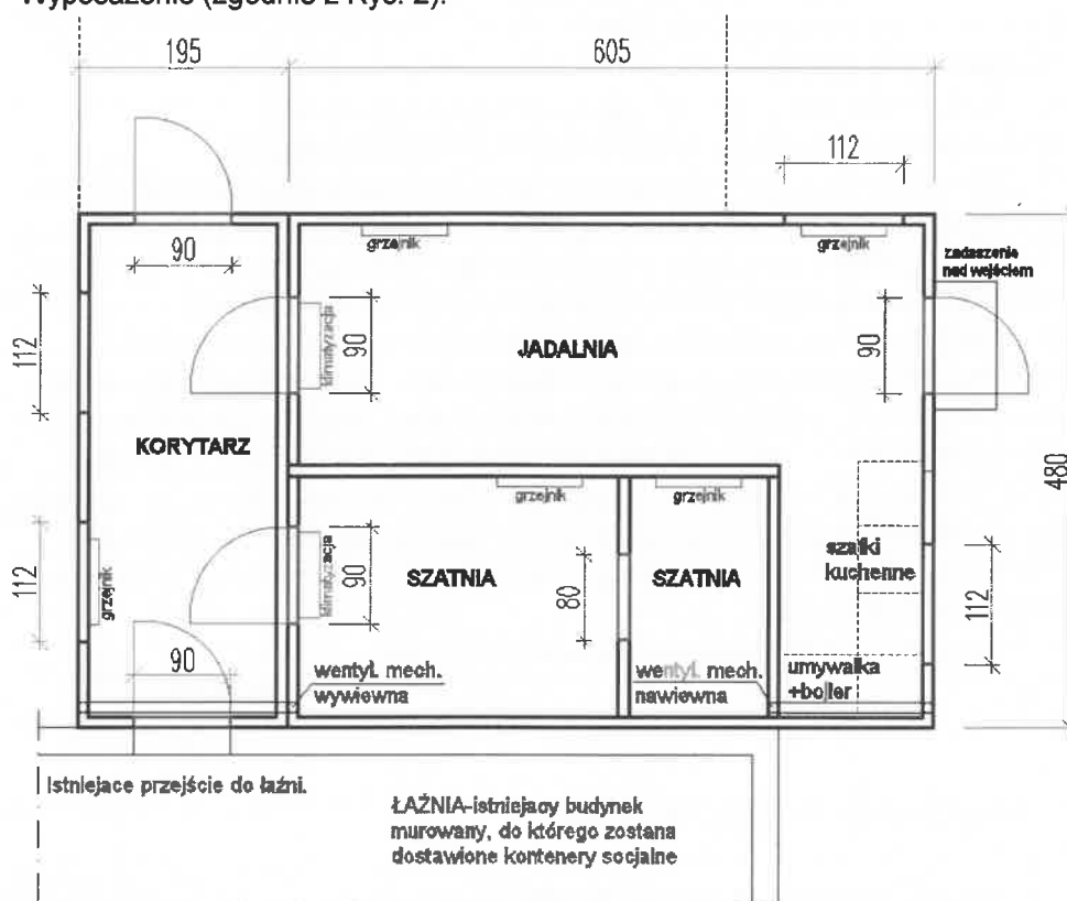
Rys. 2 Układ funkcjonalny
